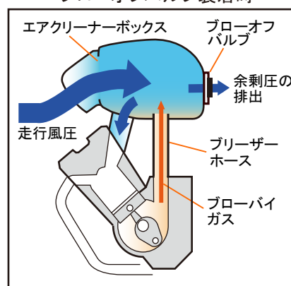
ブローオフバルブと強制減圧型NAGバルブ
