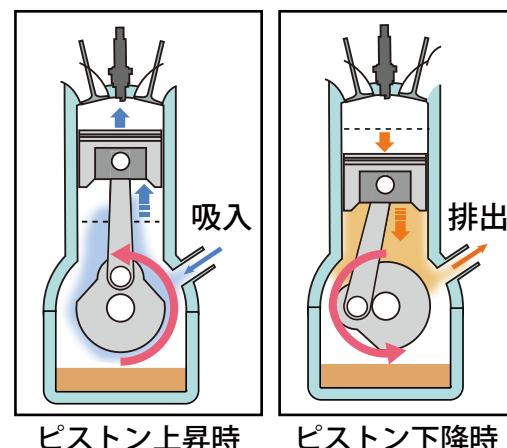
エンジン断面図
